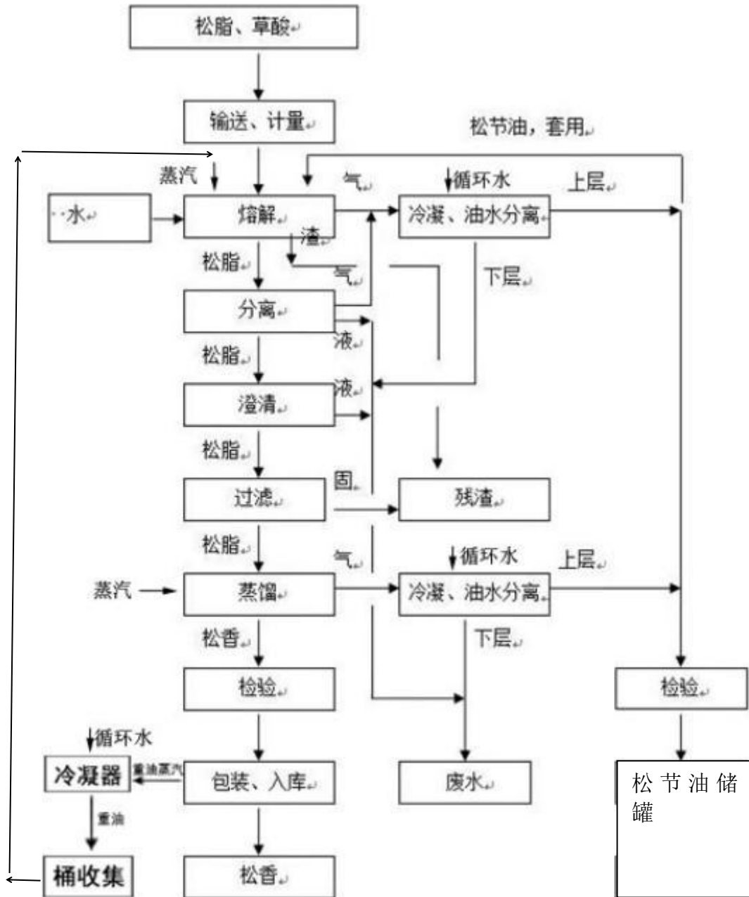
图 2.7-1 工艺流程图
